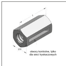
Złączka dystansowa sześciokątna (wersja z otworami kontrolnymi)
